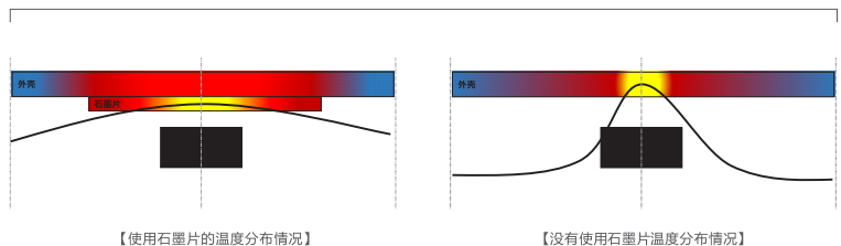
X-Y 轴方向热量传输示意图
