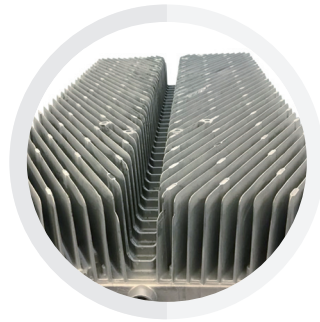
半固态压铸
